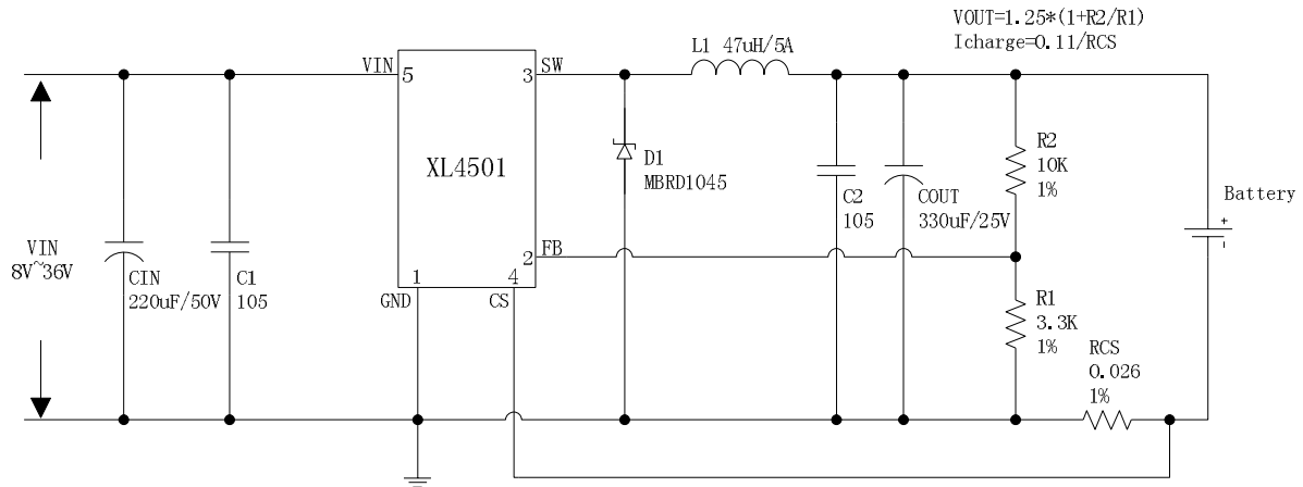
图 6. XL4501 系统参数测量电路 (VIN=8V~36V, VOUT=5V/0.1A~4.2A)
